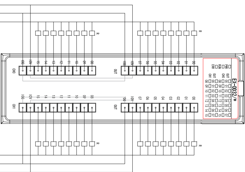
EX-OD32 EX-OD32P DO 32 points OUTPUT MODULE トランジスタ出力ユニット 32点晶体管输出单元
