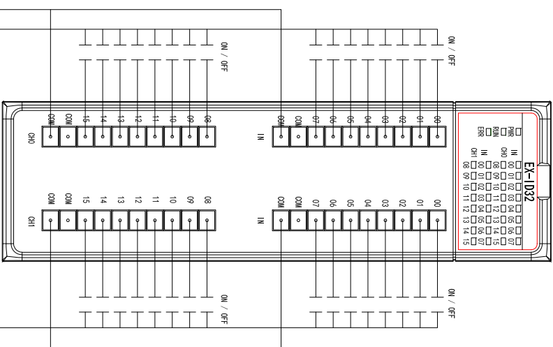
EX-ID32 DI 32 points INPUT MODULE DC入力ユニット 32点入力单元
