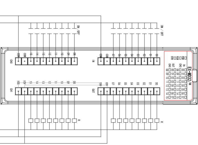
EX-MD32 EX-MD32P DI 16 points, DO 16 points MODULE 接点入出力カード (DI16、DO16) 16点輸入/16点输出单元
